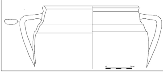
Çizim 4. InvNr.Li02-265-150 (S. Baybo – B. Yener-Marksteiner)
