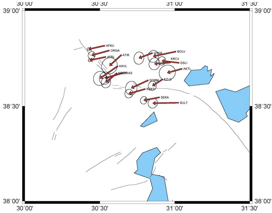
Şekil 4. Bölgenin Avrasya sabit hız alanı
