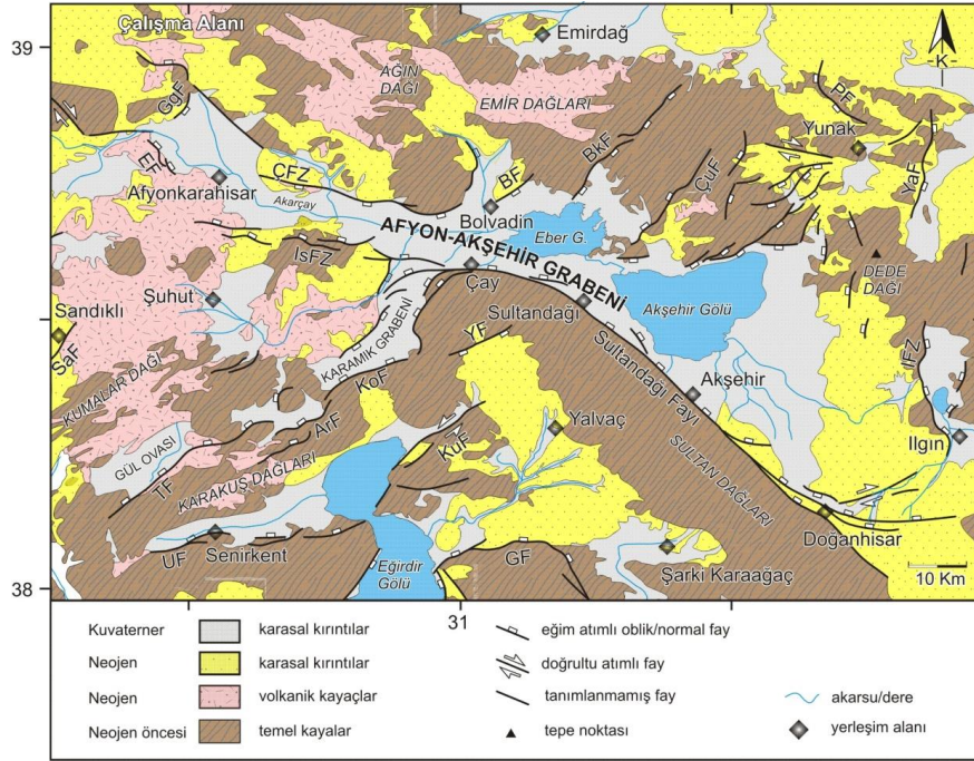
Şekil 1. Afyon-Akşehir Grabeni ve çevresinin jeoloji haritası ([7] ve [17]' den düzenlenmiştir)
