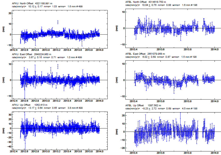
Şekil 3. AFKU ve AFBL sabit GNSS istasyonlarının günlük zaman serisi
