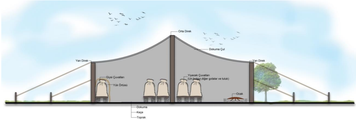
Şekil 7. Gönen Yaylası'nda tespit edilen Sarıkeçeliler'e ait kıl çadırın kesit krokisi.
