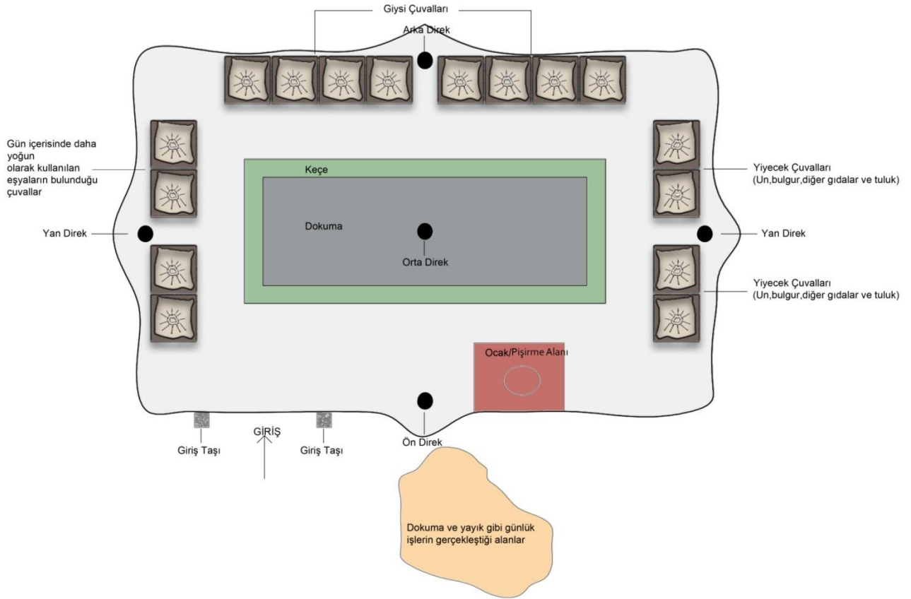
Şekil 6. Gönen Yaylası'nda tespit edilen Sarıkeçeliler'e ait kıl çadırın plan krokisi.
