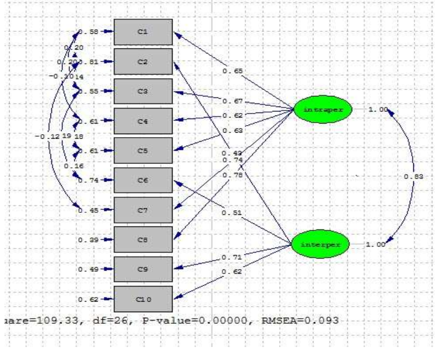
Şekil 1. Dini Bağlılık Ölçeği-Türkçe Formu'na İlişkin Path Diagramı ve Faktör Yükleri
