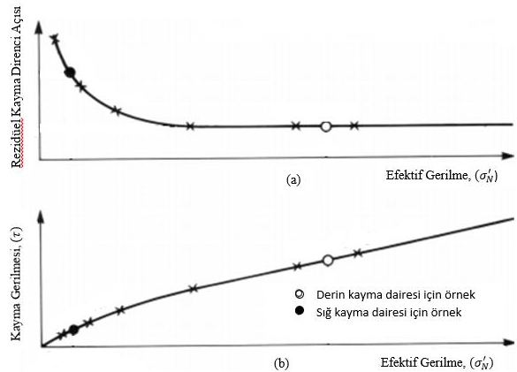
Şekil 2. Rezidüel Kayma Direnci Açısının ve Kayma Gerilmesinin Efektif Normal Gerilmeye Göre Değişimi (Variation of Residual Friction Coefficient and Shear Stress with Effective Normal Stress) [18]
